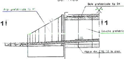
SECTIUNE 1 - 1 Sc.1:100
